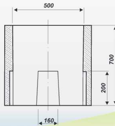
Przekrój poprzeczny
