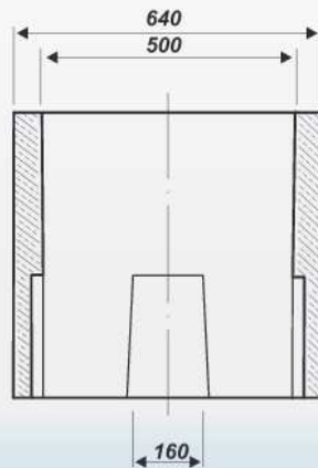
Przekrój podłużny
